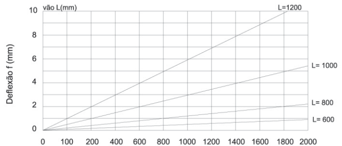
Carga p (Kg/m) DISTRIBUÍDA
